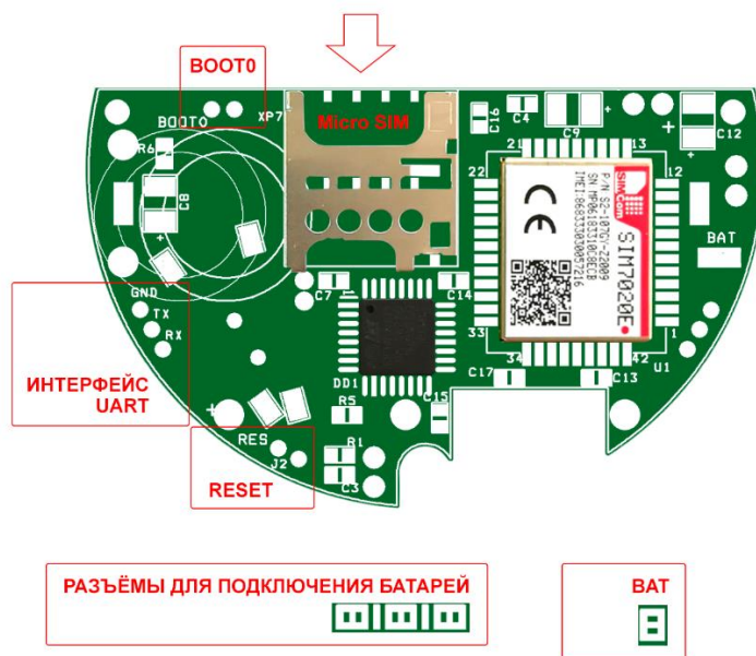
Рисунок 2 – Расположение интерфейсного разъема UART и джамперов ВАР, RESET, BOOT0 и разъёмов для подключения батарей.
